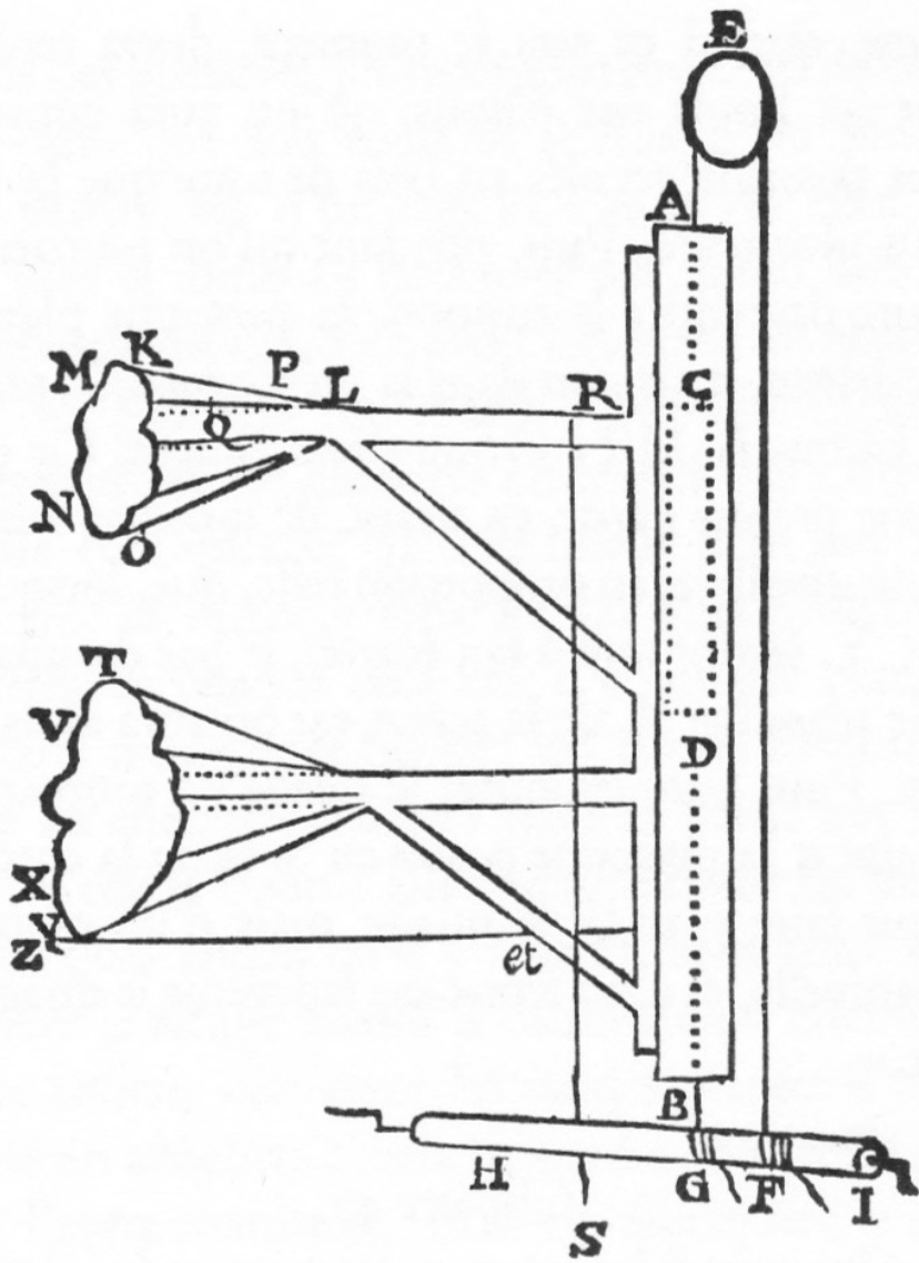
Nicola SABBATINI, Pratique pour fabriquer scènes et machines de théâtre , livre second, 1638, chap. 46 « Comment faire descendre un petit nuage qui, à mesure qu'il descend, devient toujours plus grand. »
